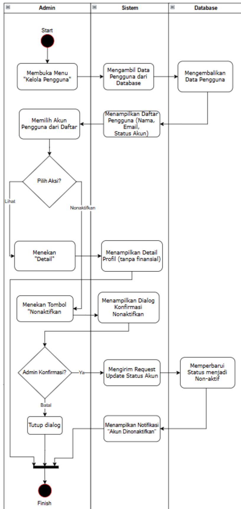
Gambar 13 Activity Diagram Admin Mengelola Pengguna
