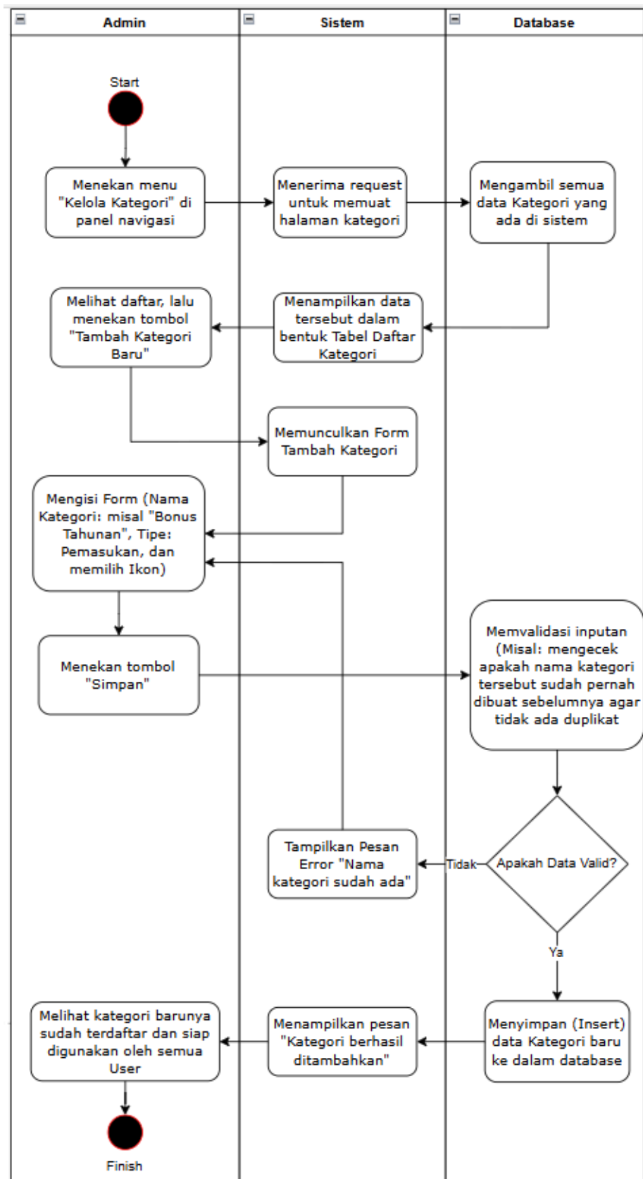
Gambar 12 Activity Diagram Admin Mengelola Kategori Transaksi
