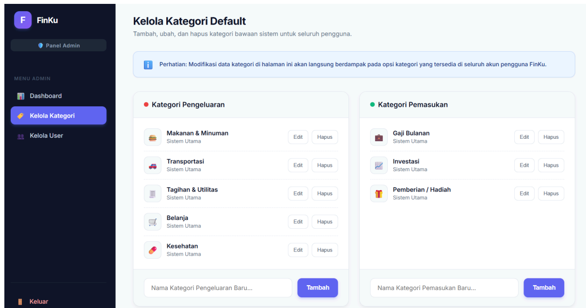
Gambar 34 System Prototype Kelola Kategori
